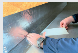
7. 10 cm-Liner abziehen
